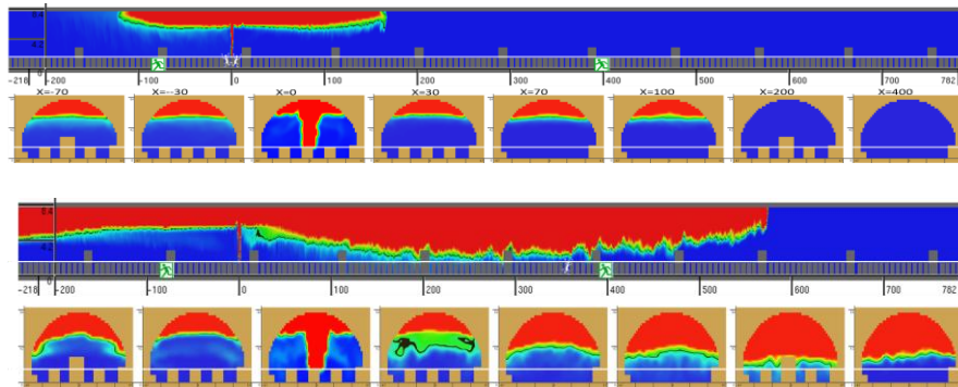
道路トンネル内火災時煙拡散・避難可否シミュレーションイメージ
