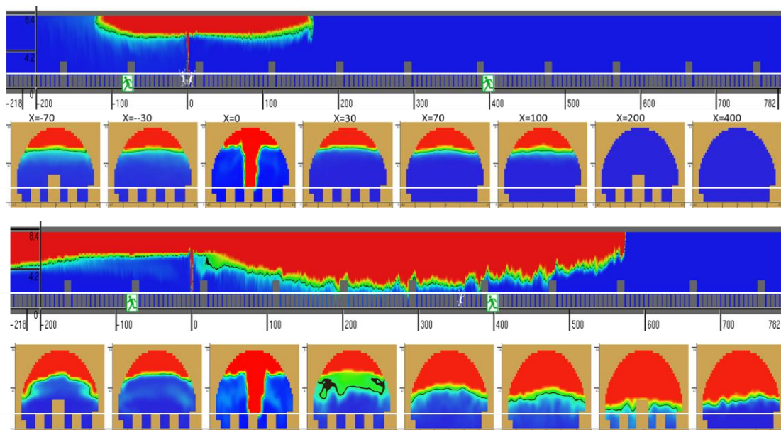
道路トンネル内火災時煙拡散・避難可否シミュレーションイメージ
